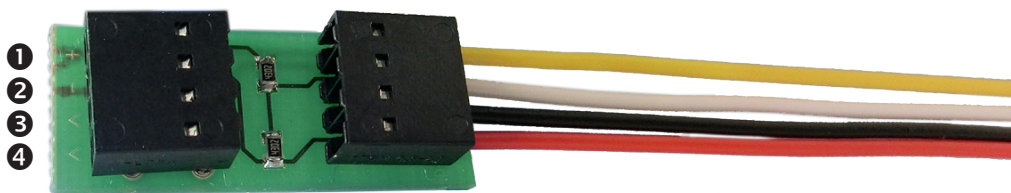
Abb. 3: Abschlussmodul AM 142
