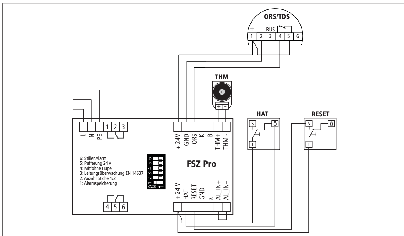
Abb. 5: Anschluss nach DIBt ohne Leitungsüberwachung
