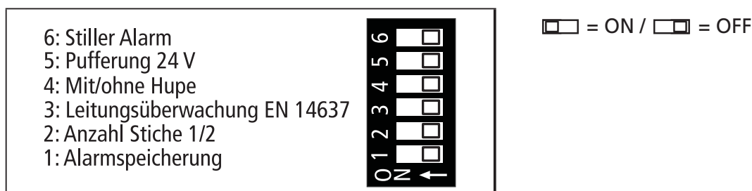
Abb. 4: DIP-Schalter für Konfiguration der FSZ Pro
