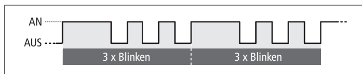
Abb. 13: Beispiel Blinksequenz 3 x Blinken
