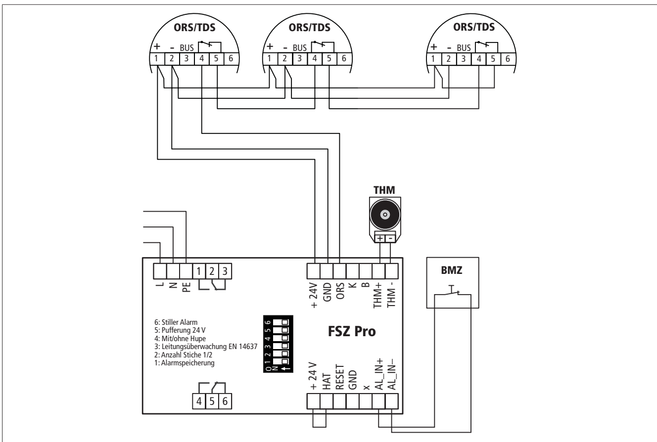
Abb. 6: Anschluss nach DIBt ohne Leitungsüberwachung
