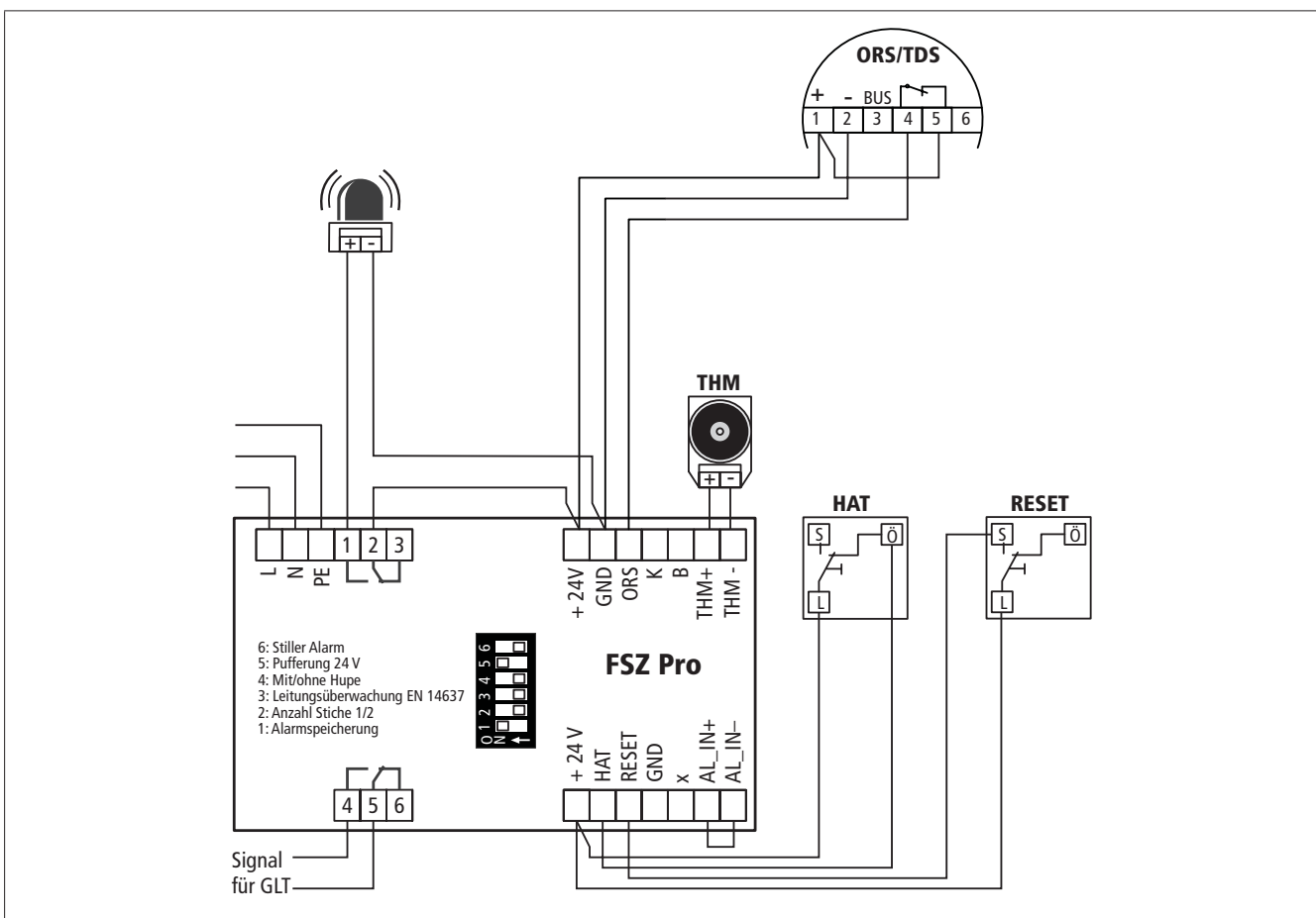
Abb. 10: Anschluss nach DIBt ohne Leitungsüberwachung
