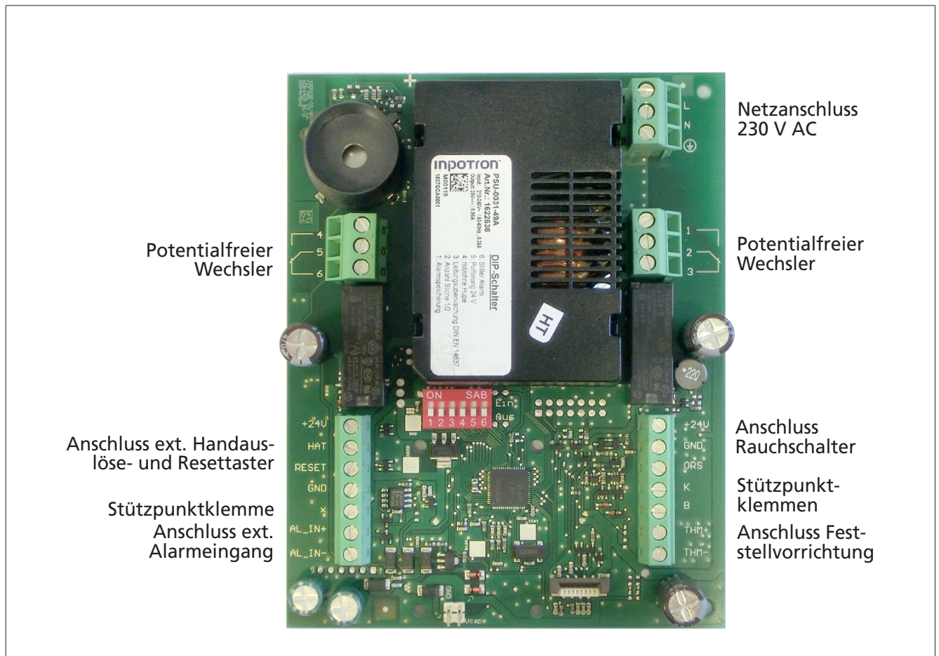
Abb. 2: Klemmenbelegung FSZ Pro
